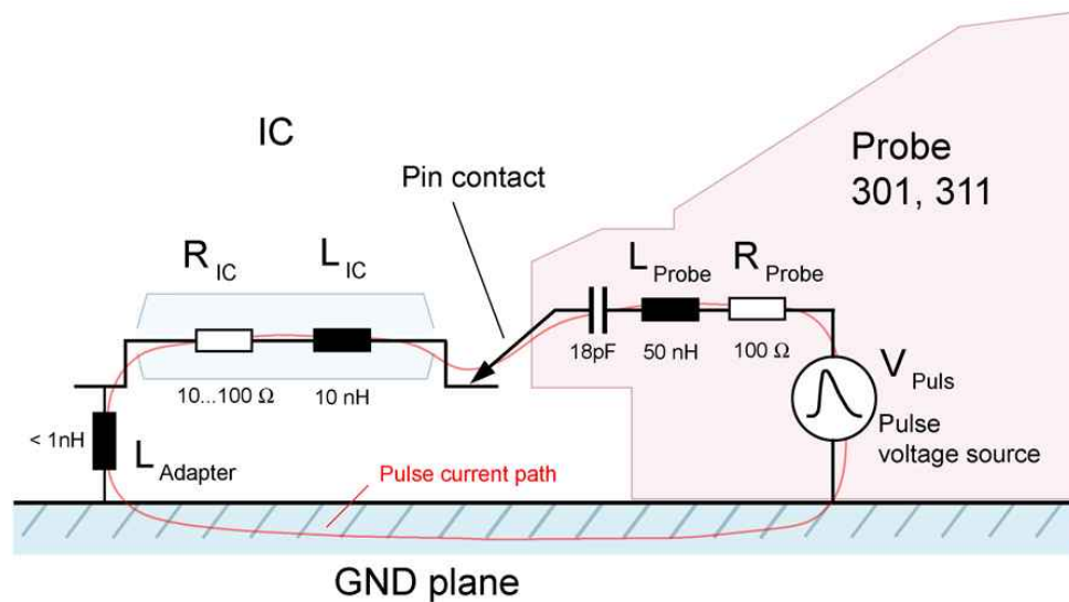
Ersatzschaltbild
