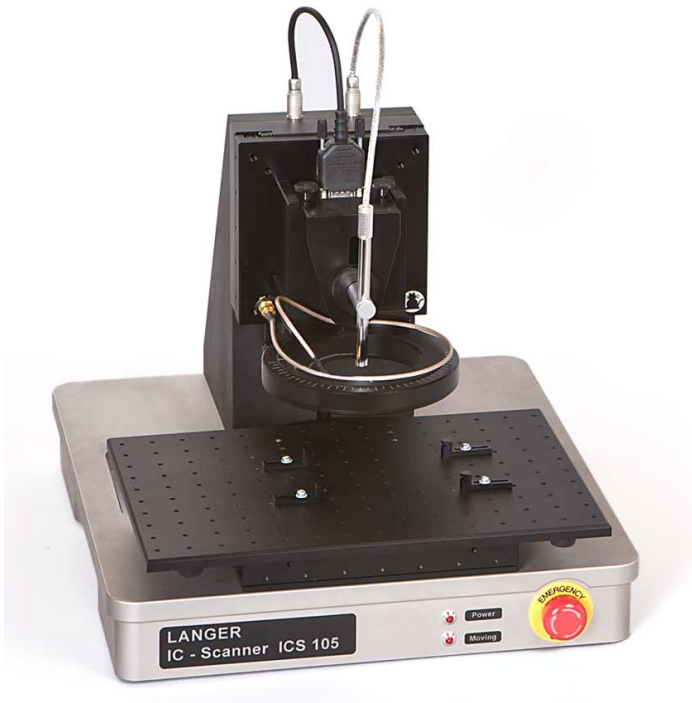
ICS 105 mit Universalhalter UH DUT und Prüfling
