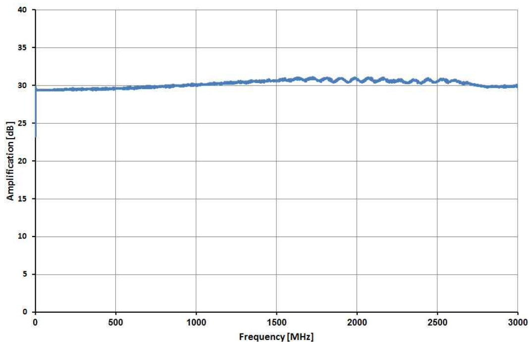
频率特性
