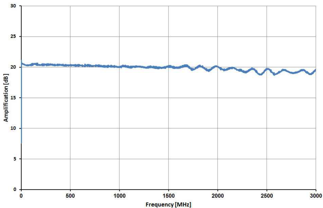
频率特性
