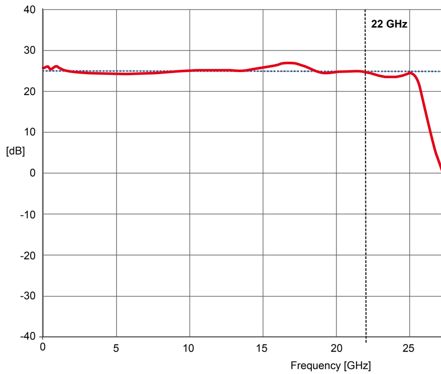
频率特性
